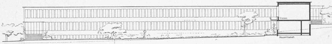
Südostfront des Schulfügel und Schnitt durch den Sing- und Vortragsaal. — Masstab 1 : 600.
