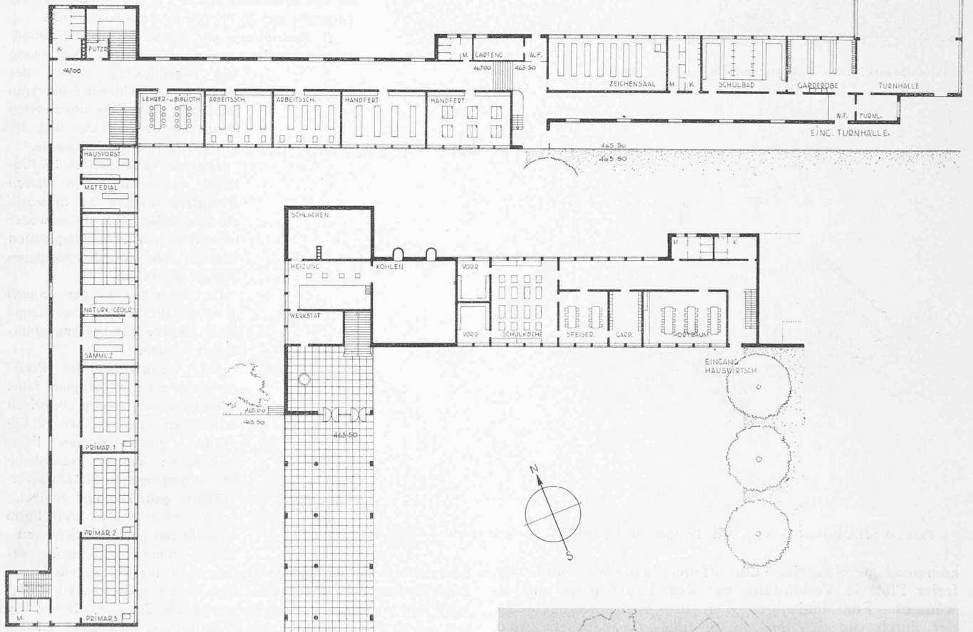
I. Obergeschoss, 1 : 600. (Im Programm vorgeschriebene Zimmergröße 10 × 6,5 m.)
