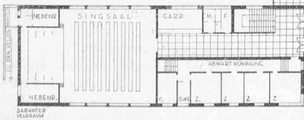
Erdgeschoss. Masstab 1 : 600. — Rechts: Isometrie 1 : 2000.
