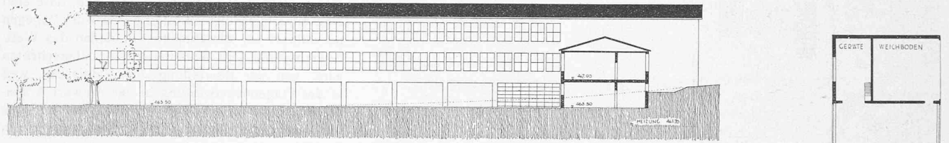
Südfassade des Schulhausflügels mit Spielhalle im Erdgeschoss. — Masstab 1 : 600.
