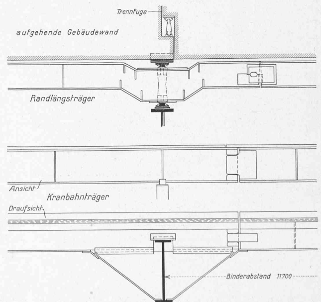
Abb. 6. Längsglieder mit Binderanschluss. — Masstab 1 : 60.
