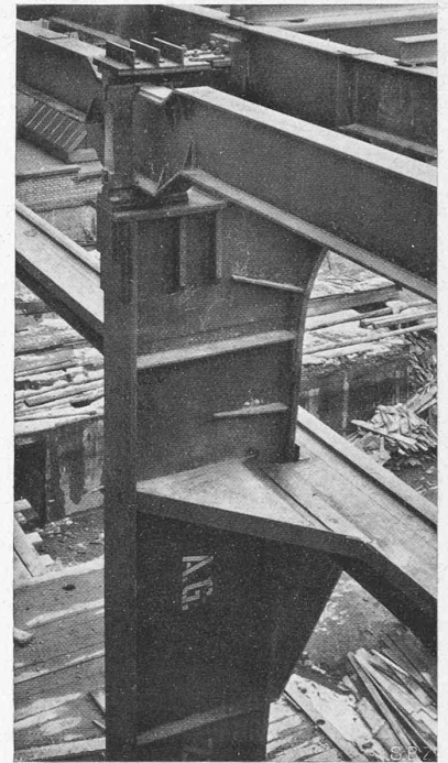
Abb. 5. Montagebild.
