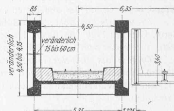
Abb. 3. Querschnitt, Masstab 1 : 200.
