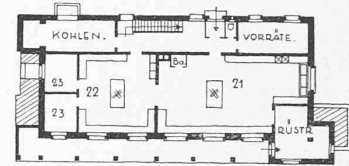
ERDGESCHOSS
