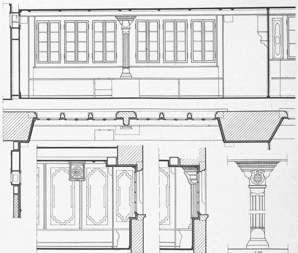
Fenstersäule, 1 : 30.
