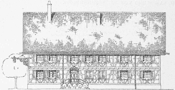
Abb. 29. Ostfront mit Haupteingang. — 1 : 300.
