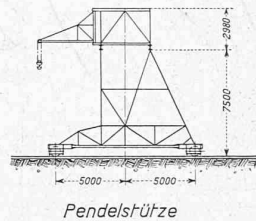
Pendelstütze
