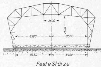
Feste Stütze
