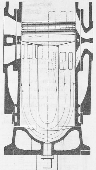
Abb. 10. Darstellung der Spülung der untern Zylinderseite. Vertikal- u. Horizontalschnitt. 1:30.
