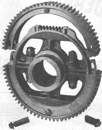
Abgedertes Maag-Traktionsrad, Type Protex (Montreux-Oberlandbahn)
