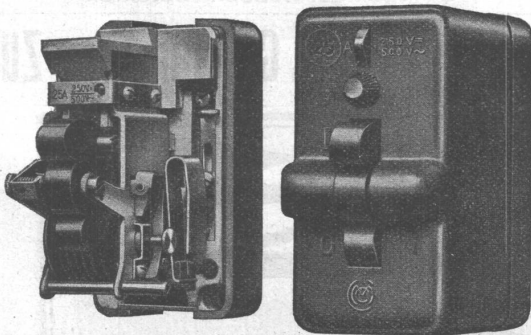
Installations-Selbstschalter 500 Volt, 25 Amp. mit Nulleiterklemme
