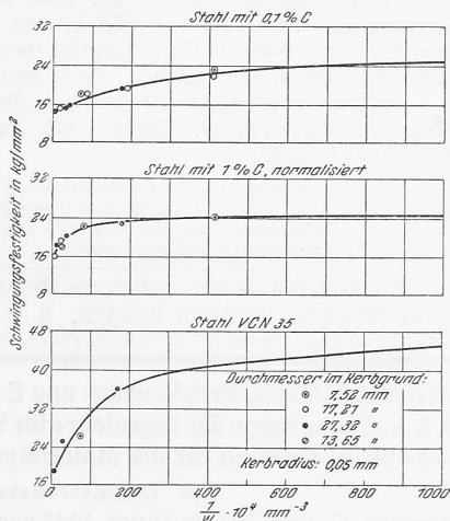
Abhängigkeit der Schwingungsfestigkeit gekerbter Stähle vom reziproken Wert des Ringwiderstandsmomentes 1/W ;
