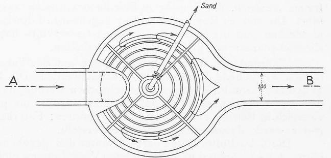
Abb. 2. Vertikal durchflossener Sandfang, Grundriss und Schnitt. — 1 : 125.
