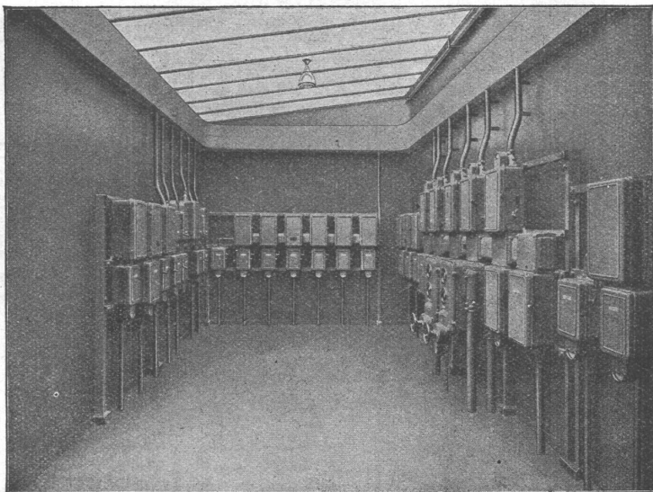
Gekapselte Niederspannungs-Anlage in einer Grossmetzgerei.
