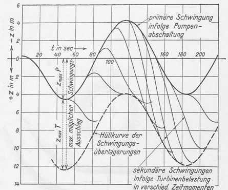
Abb. 21. Betriebsumstellung: Abschaltung von 2 Pumpen (- 32 m³/sec) und darauffolgendes Anlaufen zweier Turbinen (+ 50 m³/sec).
