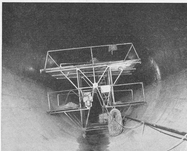
Abb. 16. Schalungsrohr fertiger Stollen mit Inertolanstrich der Kalotte. Gerüstwagen für Revision, Injektionen, Anstrich u. dgl.
