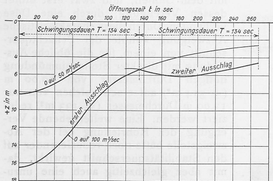
Abb. 19. Maximale Schwingungsausschläge in Funktion der Turbinen-Oeffnungszeit, für Belastung 0 auf 50, bzw. auf 100 m³/sec.
