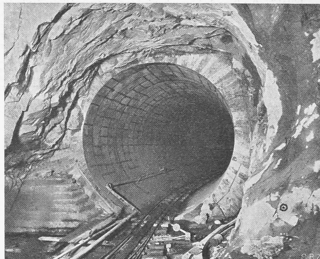
Abb. 15. Schalungsrohr betonierter Druckstollen \varnothing 5,50 m beim Wasserschloss; die dunkeln scheinbaren Fugen sind Abdruck der Eisenschalung.
