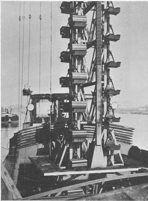
Abb. 6. Beladen der Becherkette im Rheinkahn.
