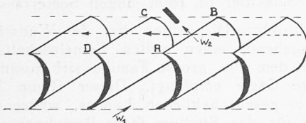
Abb. 12. Aufnahme der Gesamtdruckverteilung hinter Dampfturbinen-Schaufelreihen.
