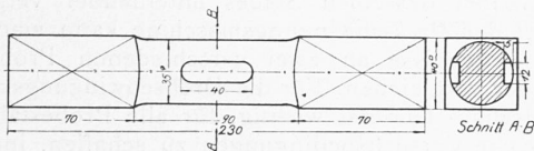
Abb. 1. Probestab für Verdrehungsversuche.
