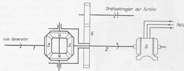
Abb. 23. Drehzahl-Reguliereinrichtung.
