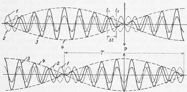
Abb. 24. Spannungsdiagramm vor der Parallelschaltung.
