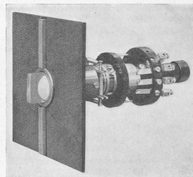
Abb. 20. Symbolschalter.
