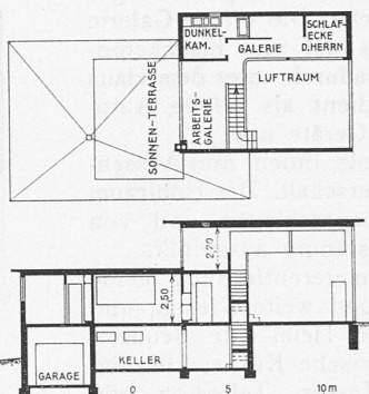
Abb. 2. Grundrisse und Schnitte 1:400.
