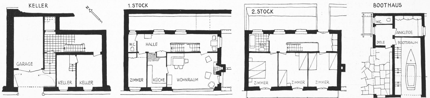
FERIENHAUS IN MORCOTE AM LUGANERSEE (noch nicht vollendet). Arch. Bräuning, Leu, Dürig in Basel.
