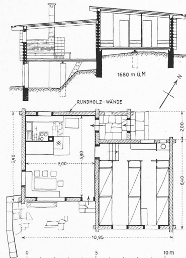
Abb. 42 Grundriss und Schnitt 1 : 250, Abb. 43 und 44 Ansicht des Blockhauses im Sertigtal bei Davos. Architekten Hans Von der Mühlhll und Paul Oberrauch, Basel. — Baukosten samt Einrichtung rd. 15 000 Fr.
