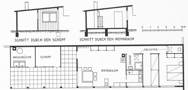
Abb. 61. Risse 1 : 250. Abb. 62. Detail 1 : 20.
