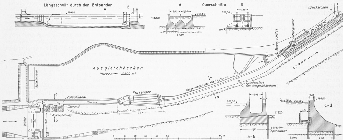
Abb. 10. Lageplan (1:1600), sowie Schnitte von Wasserfassung, Ausgleichsbecken, Dufour-Entsander und Stolleneinlauf („Druckkanal“).
