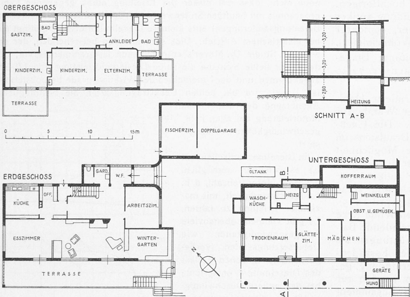
Abb. 1. Grundrisse und Schnitt des Wohnhauses am Hallwilersee. — Masstab 1 : 400.
