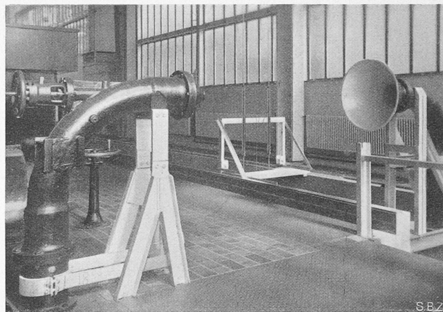
Abb. 11. Regulierbare Versuchs-Nadeldüse für Strahl bis 50 mm \varnothing und 40 m/sec. Rechts Strahl-Auffangtrichter, im Hintergrund Stechpegel des Messkanals.
