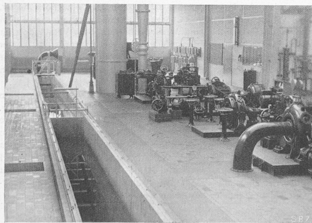
Abb. 16. Der Messkanal.
