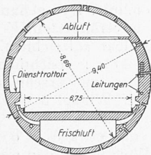
Querschnitte 1 : 300. Abb. 2. Gusseisenring-Profil des Schildvortriebes.
