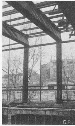
Abb. 29. Hallenbinder-Pendelstützen.
