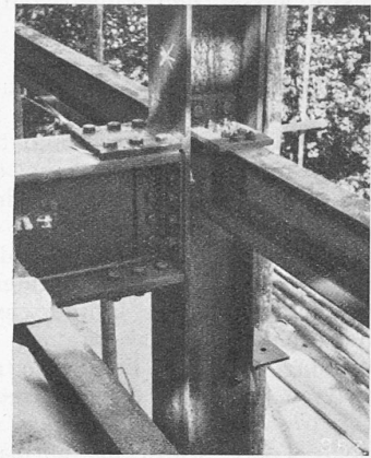
Abb. 30. Stahlskelett-Knotenpunkt.
