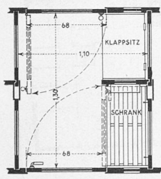
Abb. 12. Umkle-Kabine, 1 : 40.
