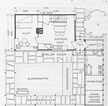
4. Preis ex aequo (300 Fr.), Entwurf Nr. 355. Verfasser M. Piccard, Arch., Zürich-Lausanne.
