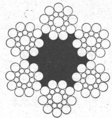
Seale- Konstruktion
