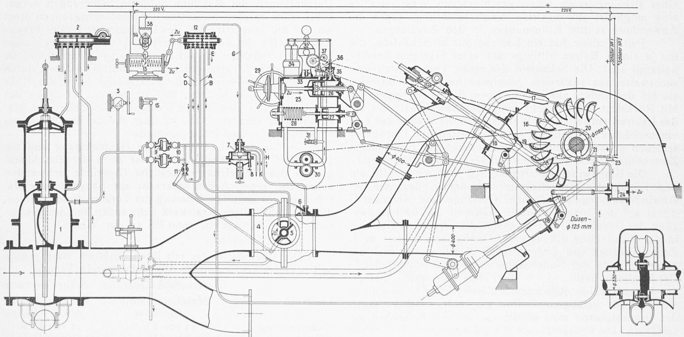
Abb. 49. Sernf-Turbine, schematisiert. Schnitt des Löffelrades (rechts) 1: 60. — Legende: 1 Absperrschieber, 2 Steuerventil des Absperrschleiers, 3 Antrieb des Schleiers für die Bremse, 4 Kugelschieber, 5 Antriebsflügel, 6 Dichtungsring, 7 Steuerautomat, 8 Regulierstift für Schliesszeit, 9 Filter, 10 Absperrventile zur Filteranlage, 11 Drosselapparat, 12 Steuerventil des Kugelschiebers, 13 Doppelhubmagnet, 14 Schalter mit selbstätiger Nullstellung, 15 Antrieb des Spülschiebers, 16 Laufband, 17 Bremsdüse, 18 Düsen, 19 Ablenker, 20 Maximalregulator, 21 Ausklinkhebel, 22 Ventil des Maximalregulators, 23 Schalter, 24 Servomotor des Maximalregulators, 25 Oeldruckregulator, 26 Nadel-Servomotor, 27 Ablenker-Servomotor, 28 Feder zum Ablenker, 29 Handregulierung, 30 Zahnradpumpe, 31 Sicherheits-Ventil, 32 Zentrifugalpendel, 33 Drehzahl-Verstellung, 34 Rückführung, 35 Nadel-Steuerventil, 36 Ablenker-Steuerventil, 37 Sicherheitsvorrichtung bei Riemenabfall, 38 Schutzwiderstand. Leitungen: A Druckleitung, B Öffnungsleitung, C Schliessleitung, D Verbindg. Ablaufleitung mit Automat, E Ablauf v. Steuerapparat, G Verbindungs-Druckleitung, H Zuleitung, I Ablauf v. Automat, K Ablauf v. Dichtungsring.
