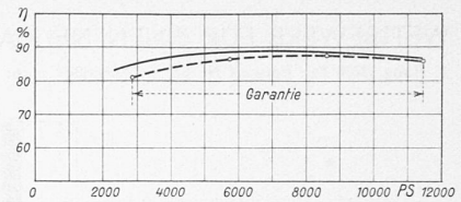
Abb. 54. Wirkungsgrade der Niederentbachturbine.
