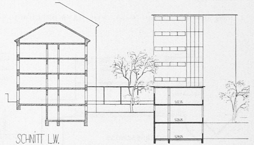
2. Rang ex aequo (3000 Fr.), Entwurf Nr. 79. Verf. OTTO HÄNNI, Arch., Zürich.
