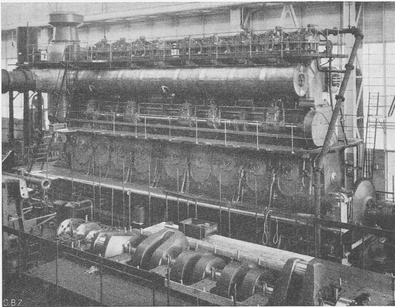
Abb. 1 (links). Einfachwirkender Sulzer-Zweitakt-Schiffsmotor, 6000 PS e , 120 U/min. — Abb. 2 (rechts). Manöverstand eines Zweitakt-Schiffsmotors, 6000 PS e , 120 U/min. 1 Umsteuerhebel, 2 Maschinentelegraph, 3 Tachometer, 4 Hebel für „Anlassen“, „Betrieb“ und „Abstellen“, 5 Hebel mit Feineinstellung zum Regulieren der Brennstoffmenge
