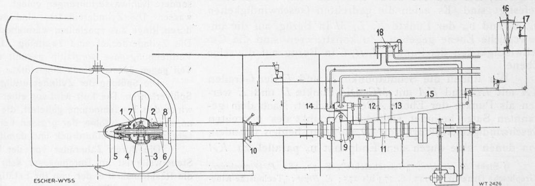
Abb. 4. Schematische Darstellung der Steuerung des Verstellpropellers beim Motorboot „Etzel“. (Legende im Text.)
