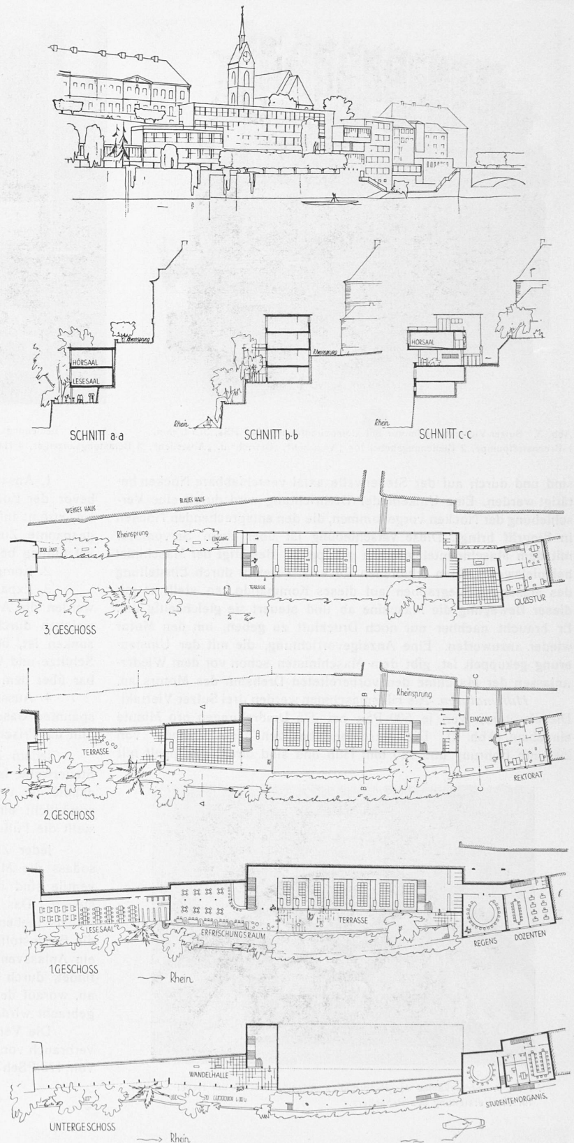
Abb. 3 und 4. Grundrisse und Schnitte 1 : 1200, sowie Perspektive des neuen Kollegengebäudes am Rhein der Universität Basel, gemäss Vorschlag der B. S. A.-Ortsgruppe Basel.
