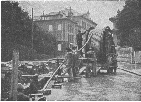
Verlegung von 6 kV Kabeln 3 x 240 mm 2 für das Elektrizitätswerk der Stadt Bern. Kabelgewicht ca. 100 000 kg.
