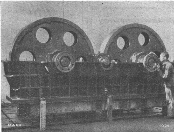
MAAG-GETRIEBE MIT GESCHLIFFENER SCHRAUBENVERZÄHNUNG zwischen Dampfturbine und zwei Generatoren in Zuckerfabrik bei Paris (3900 PS bei 59 5/600 U/min.).
