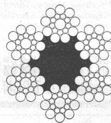
Seale- Konstruktion
