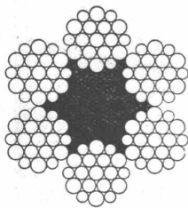
Warrington- Konstruktion
