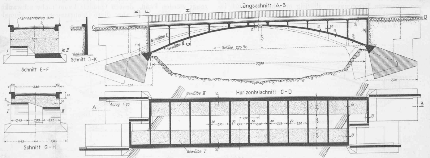
Abb. 5. Spitalbrücke über die Engstligen, Versteifter Zwilling-Stabbogen. Erbaut 1931. (Punktiert Ansichtsf lächen.) — Masstab 1 : 300.
