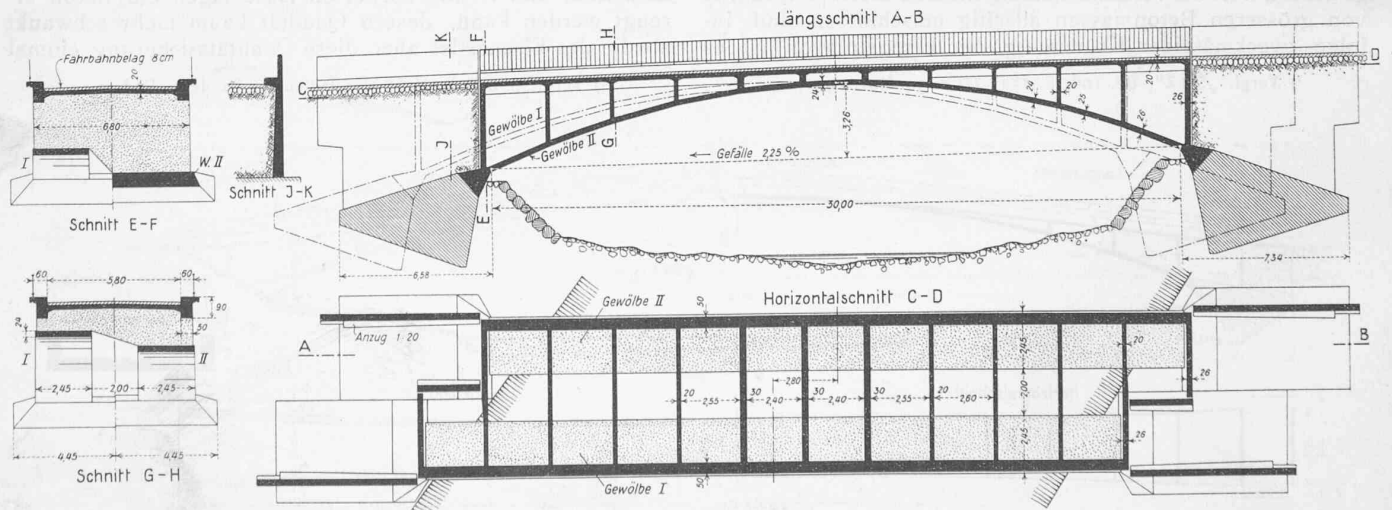
Abb. 5. Spitalbrücke über die Engstligen, Versteifter Zwillings-Stabbogen. Erbaut 1931. (Punktiert Ansichtsfächen.) — Masstab 1 : 300.
