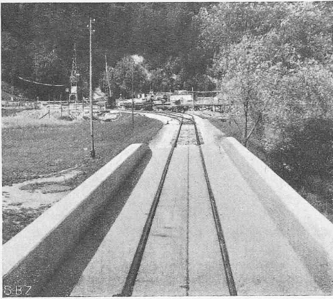
Abb. 17. Einbetoniertes Normalspurgeleise.
