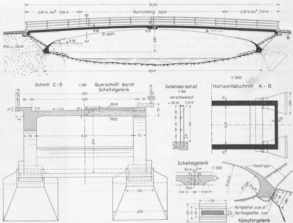
Abb. 8. Aarebrücke Innertkirchen. Dreigelenkbogen mit exzentrischer Drucklinie. Erbaut 1934. Bauzeit 4 Monate, Baukosten 162 Fr./m 2 Oberfläche. — Masstäbe 1 : 300, 1 : 120 und 1 : 60.
