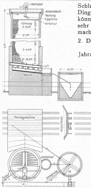
Abb. 7. Tropfkörperanlage, 1 : 100.
