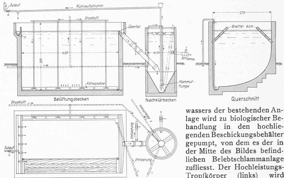
Abb. 4. Schlammbelebungsanlage, 1:100.
