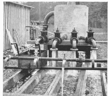
Abb. 3. Versuchsrippen mit Beschickung.
