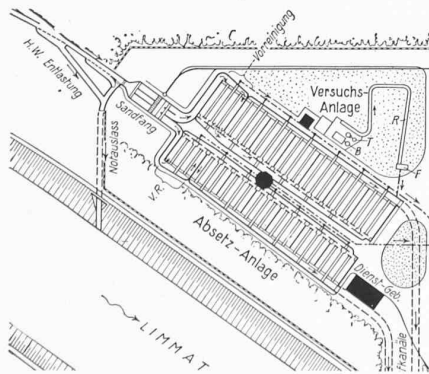
Abb. 1. Die Versuchsanlage zur biolog. Reinigung des Abwassers in der Kläranlage der Stadt Zürich. B Belebtschlammanlage, T Tropfkörper, R Versuchsrippen, F Fischteich. Masstab 1:3000.
