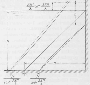
Fig. 12. Clapotis par profondeur finie.
