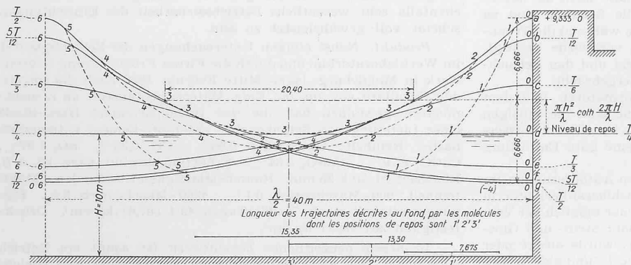
Fig. 11. Clapotis par profondeur finie. Solution de M. Sainflou : profils de la surface aux instants 0, T/12, . . . . T/2 (—) et trajectoires des particules (-----). Houle incidente : \lambda = 80 m, h = 6,66 m, H = 10 m.
