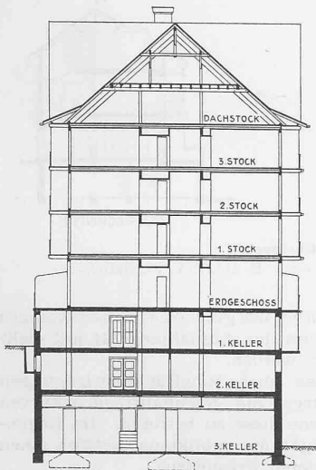
Abb. 3. Querschnitt 1: 400.
