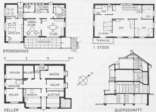
Pfarrhaus mit Amtszimmer in Rheineck . Risse 1 : 400 und Südansicht. — Arch. E. HÄNNY, St. Gallen.
