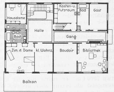
Obergeschoss
