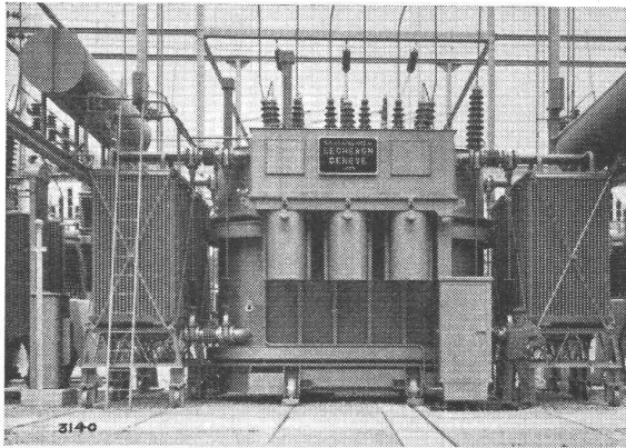
ENTREPRISES ELECTRIQUES FRIBOURGEOISES Freiluft-Transformator-Station Hauterive. — Drei- phasen-Transformator 22000 kVA, 127 auf 61 \pm 10 \times 0,9 KV, 50 Pér., mit Stufenschalter unter Last; natür- liche Oelkühlung.
