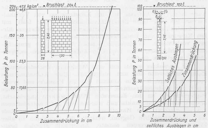
Abb. 2. Prüfung eines Novadom-Mauerwerkkörpers durch die EMPA, Zürich. — 12 Schichten, horizontale Fugen 1 cm Heraklith, vertikal Pressfugen ohne Einlage. Links zentrischer, rechts exzentrischer Druck. Druckfestigkeit der einzelnen Steine 152 bis 203 kg/cm 2 (bezogen auf den ganzen Querschnitt).
