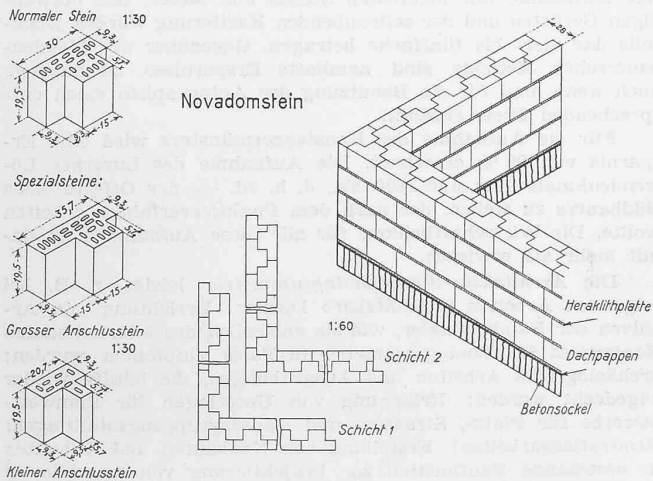
Abb. 1. Novadomstein der Ziegelei Keller & Cie., Pfungen.
