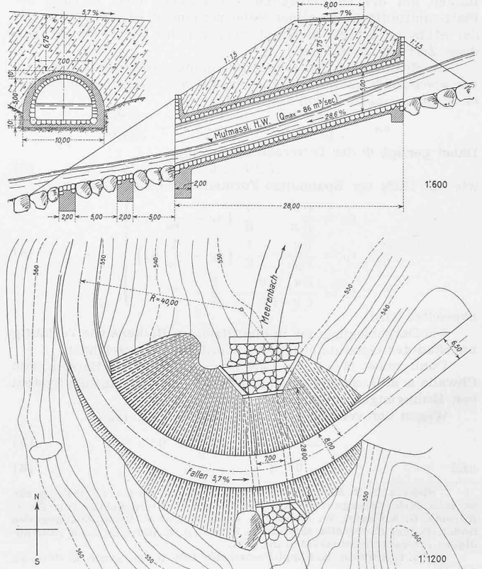
Abb. 3. Durchlass von 30 m 2 durch den Damm im Meerenbachtobel hinter Mühlehorn (Deponie des Ausbruchs aus dem Fuchsfallenhorn-Tunnel).
