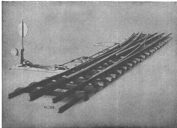
Zahnstangenweiche Jungfraubahn.
