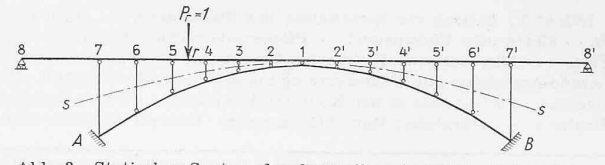
Abb. 3. Statisches System der Gesamtkonstruktion; äusserlich 5-fach, innerlich 13-fach unbestimmt.
