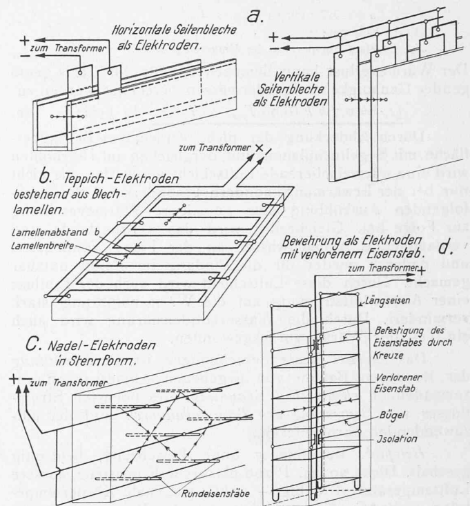
Abb. 3. Verschiedene Elektrodenarten: a) Volumenerwärmung mit horizontalen und vertikalen Seitenblechen; b) Oberflächenerwärmung mit Elektrodenteppich; c) Nadelenerwärmung mit eingesteckten Abfallrundeisen; d) Bewehrungserwärmung mit verlorenem Eisenstab.
