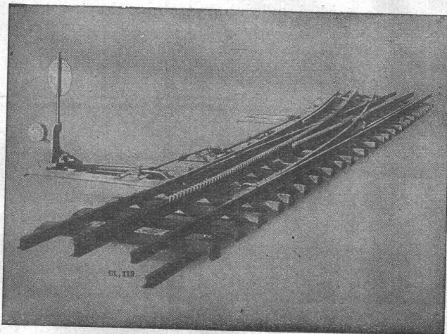
Zahnstangenweiche Jungfraubahn.
