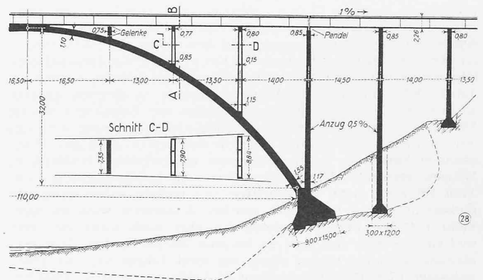
5. Rang (3000 Fr.), Entwurf Nr. 28. Ingenieurbureau BUSS A. G., Basel mit Arch. H. BAUR, Basel.
