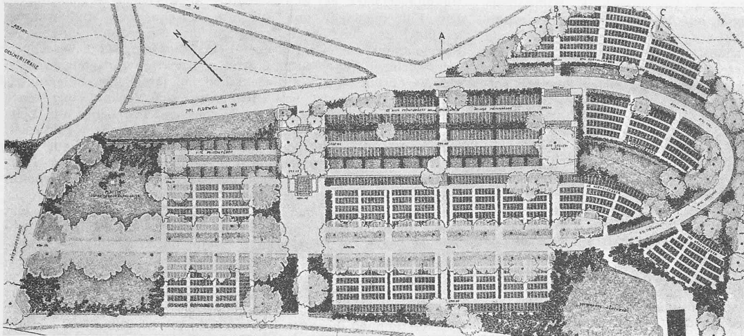
2. Rang «Pietät». Plan 1 : 1500, Profile 1 : 800. Architekt H. BEGERT, Zollikon.
