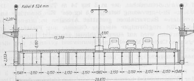
Abb. 3. Querschnitt 1: 400 der Triborough Bridge.
