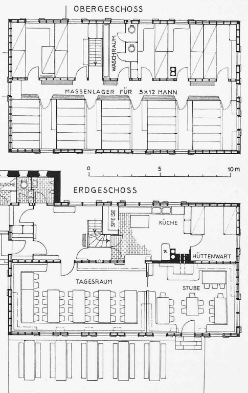
Abb. 3 (oben). Grundrisse und Schnitt. — Masstab 1:250.
