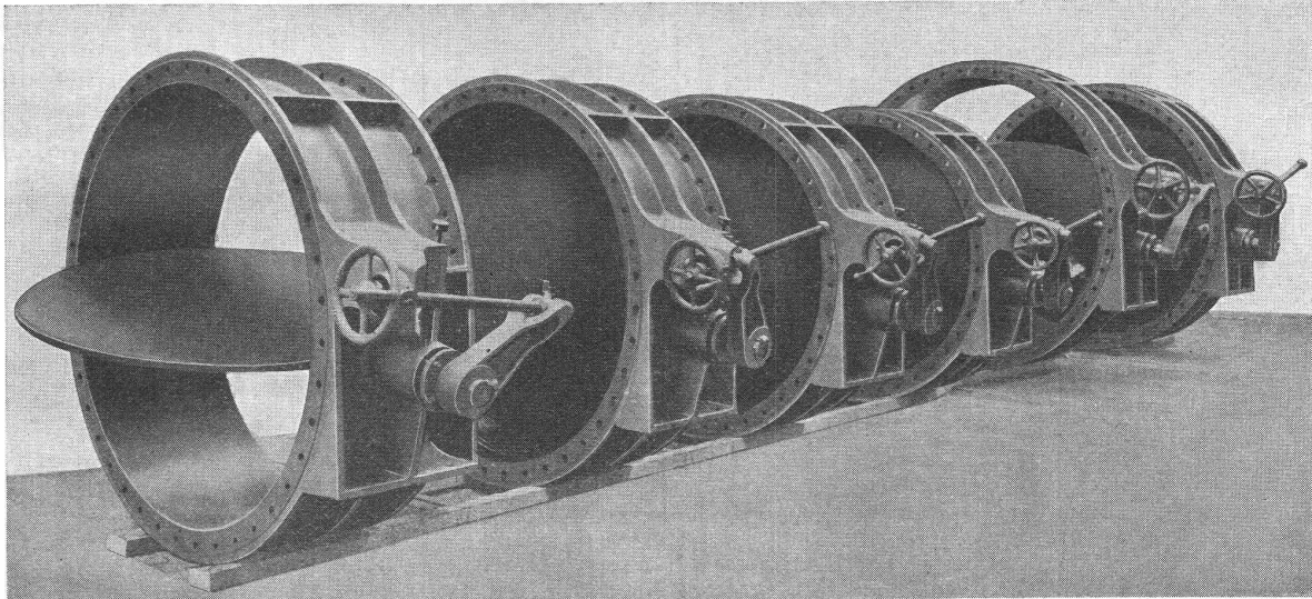
6 Drosselklappen von 2000 und 1600 mm Nennweite und 0,6 at Druck zu einer Pumptanlage in Egypten.
