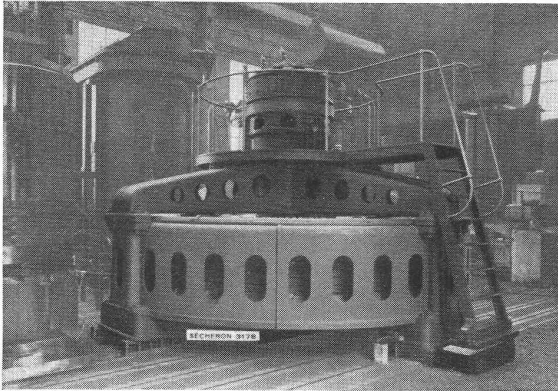
A.-G. ELEKTRIZITÄTWERKE WYNAU, LANGENTHAL. Ausbau des Werkes Wynau. Dreiphasen Generator 2000 kVA, 9500 V, 50 Per : Sek, 125 T : Min. GD 3 150000 kgm 2 zum Antrieb durch eine Kap- lanturbine (zwei Einheiten werden z. Zt. montiert). Im Kraftwerk Wynau sind schon zwei Sécheron Generatoren 1500 k VA bei 125 T : Min im Betrieb.
