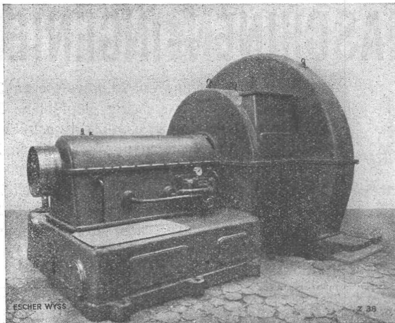
Kontinuierlich arbeitende Schub-Zentrifuge mit 1300 mm Trommel- durchmesser. Leistung: 5 Tonnen zentrifugiertes Verdampfersalz je Stunde.
